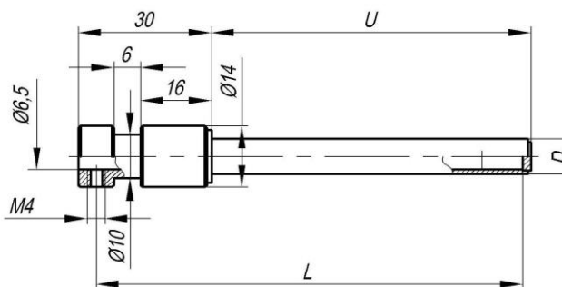
Рисунок В.4 — Гильза защитная ЮНКЖ 012
