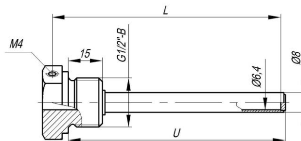
Рисунок В.3 — Гильза защитная ЮНКЖ 011—Б
