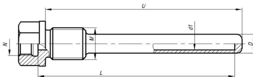
Рисунок В.9 — Гильза защитная ЮНКЖ 014 для установки термопреобразователя с подвижным штуцером
