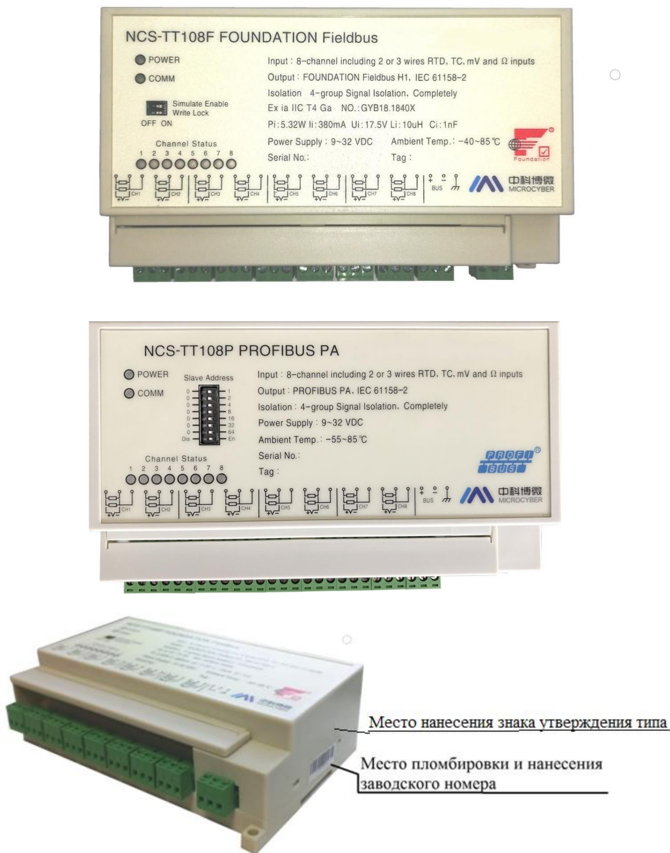
Рисунок 6 – Общий вид преобразователей измерительных NCS-TT108F, NCS-TT108P
